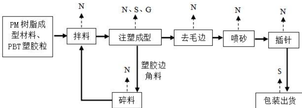
图 3-2 项目变压器骨架生产工艺及产污环节图
