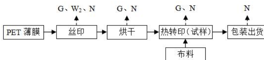
图 3-4 项目烫画生产工艺及产污环节流程图
